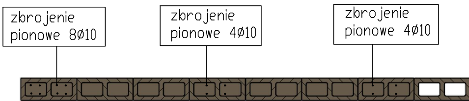
PRZEKRÓJ A-A SKALA 1 : 20
