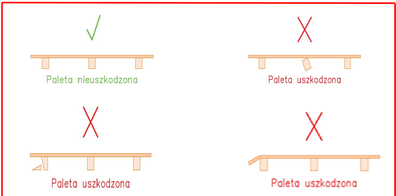
Rys. 3 Rzuty boczne
