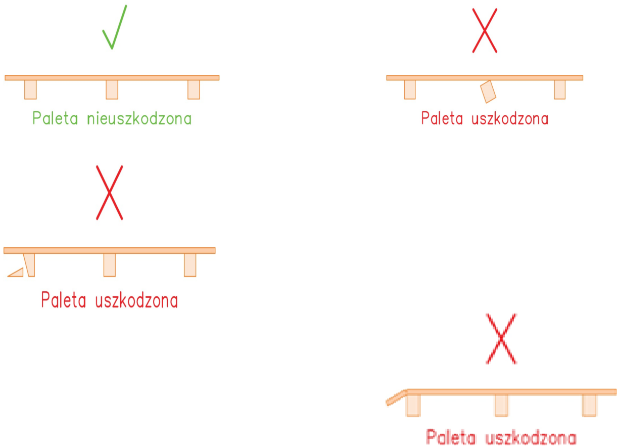
Rys. 3 Rzuty boczne
