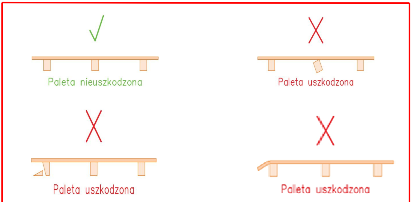
Rys. 3 Rzuty boczne
