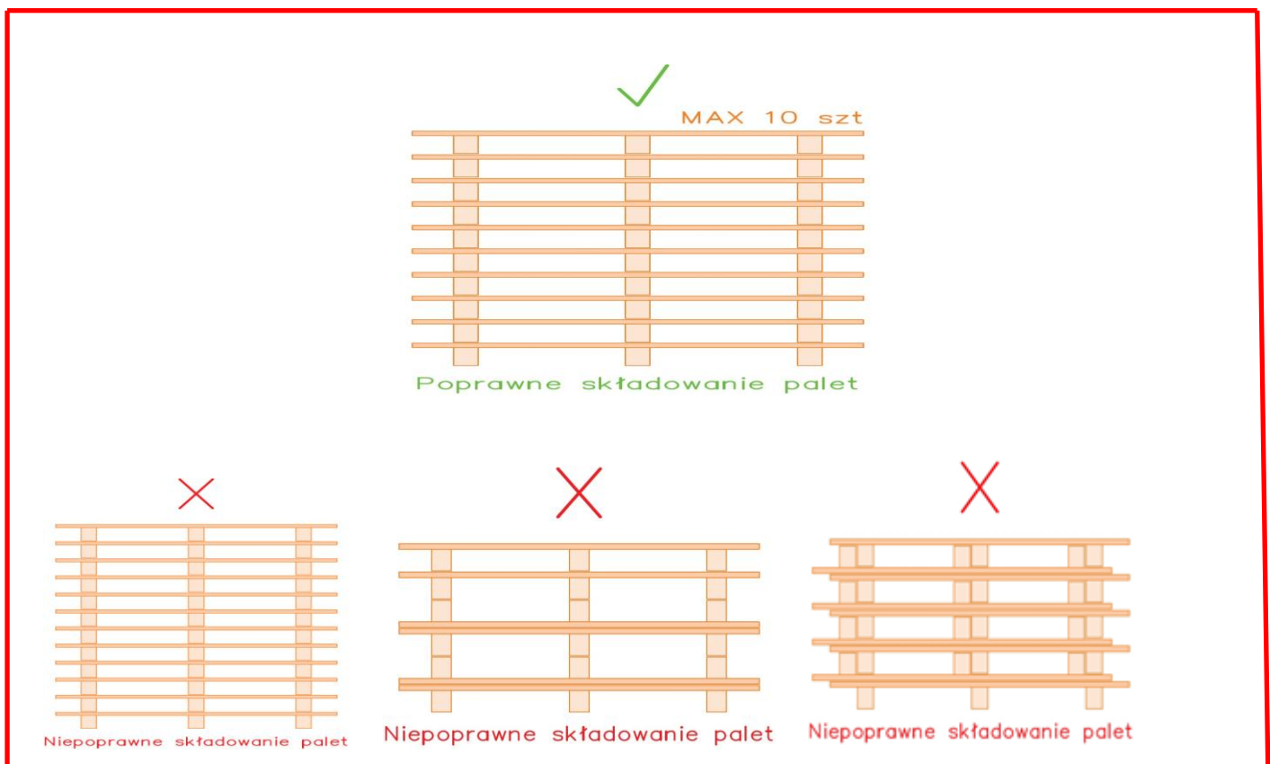
Rys. 1. Rzuty boczne
